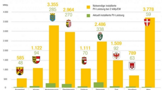
INSTALLIERTE PV-LEISTUNG PRO BUNDESLAND UND NOTWENDIGE INSTALLIERTE LEISTUNG BEI 2 KWP/EINWOHNER
